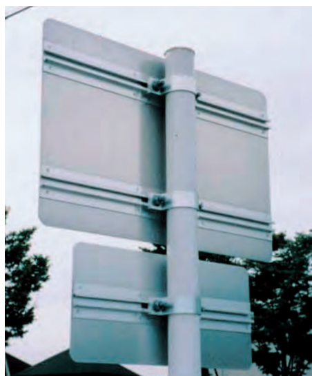
標識板 3 (既製材→アルミ板・平リブ・Uバンド・ 60.5 φ ポール使用)
